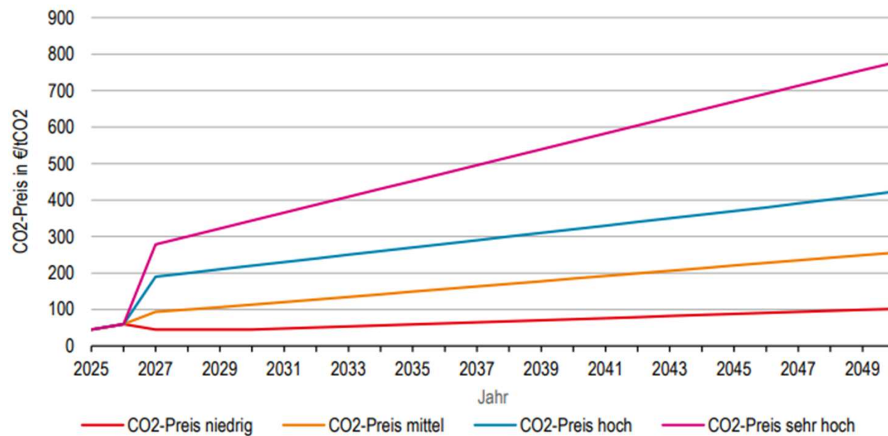
Abbildung 1: CO 2 -Preis-Projektionen
